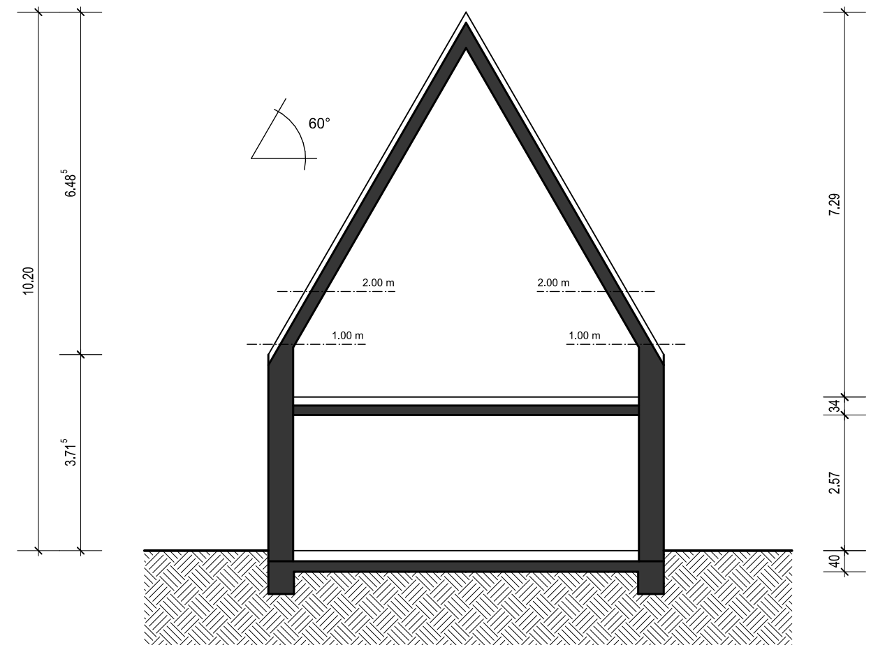
Schnitt B - B Stiftshaus
