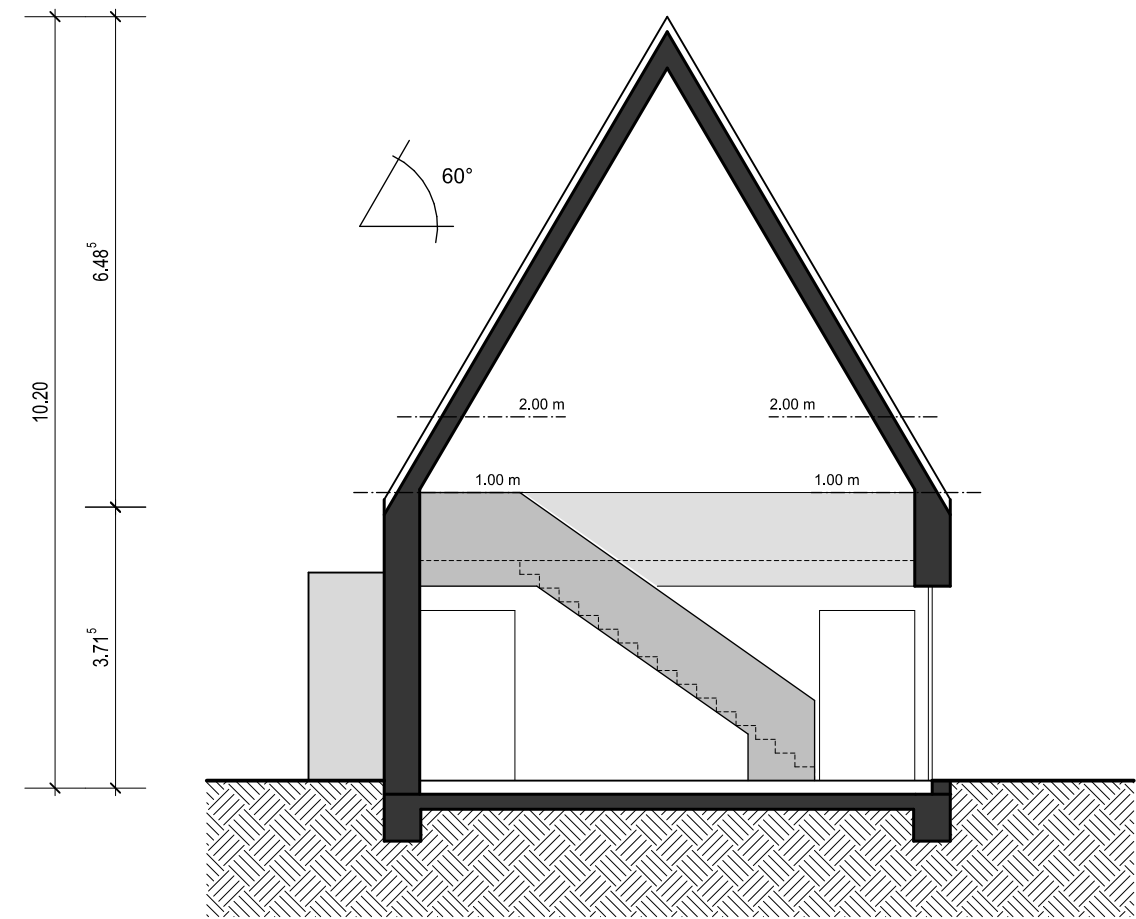
Schnitt A - A Stiftshaus
